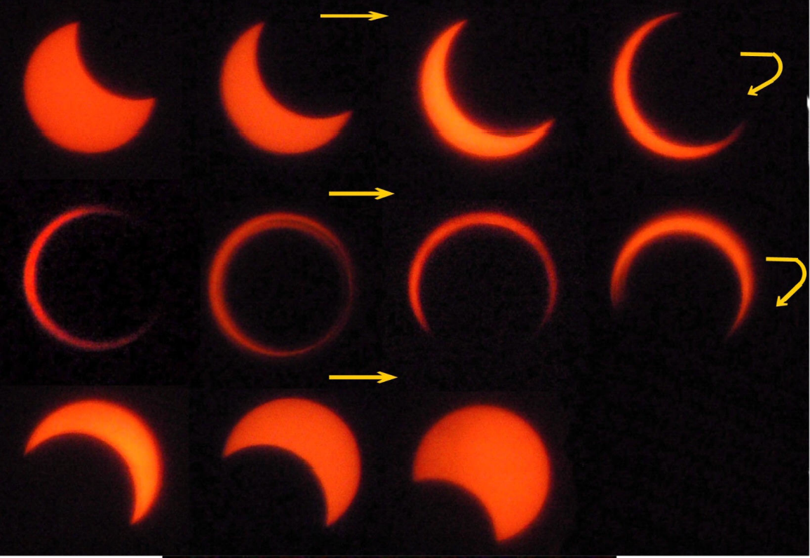
平成24年5月21日(月) 金環日食
