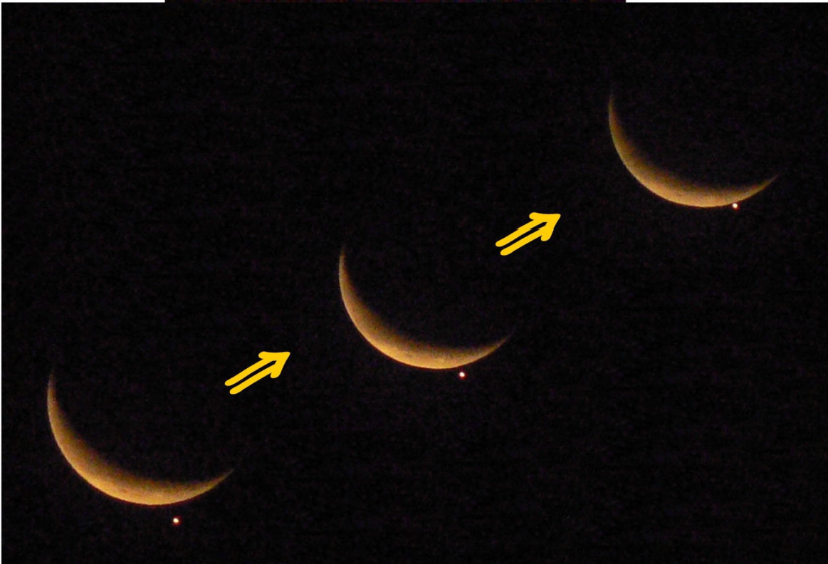
平成24年8月14日(火) 月による金星食
